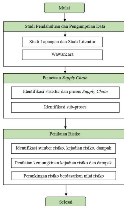
Gambar 1. Metodologi penelitian
